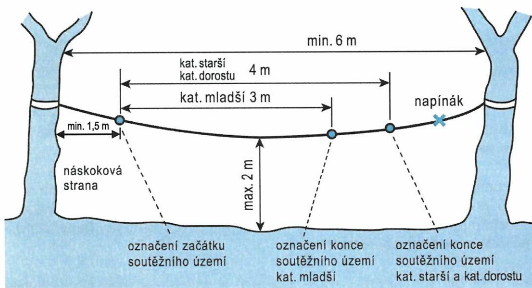
Obr. 5 Brannost - Náskres stanoviště překonání překážky po vodorovném laně
